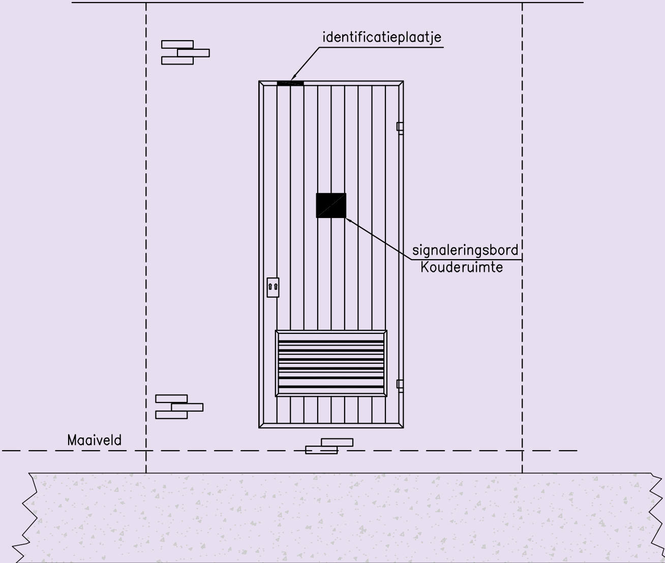
Voorraanzicht gevel (A-A)
