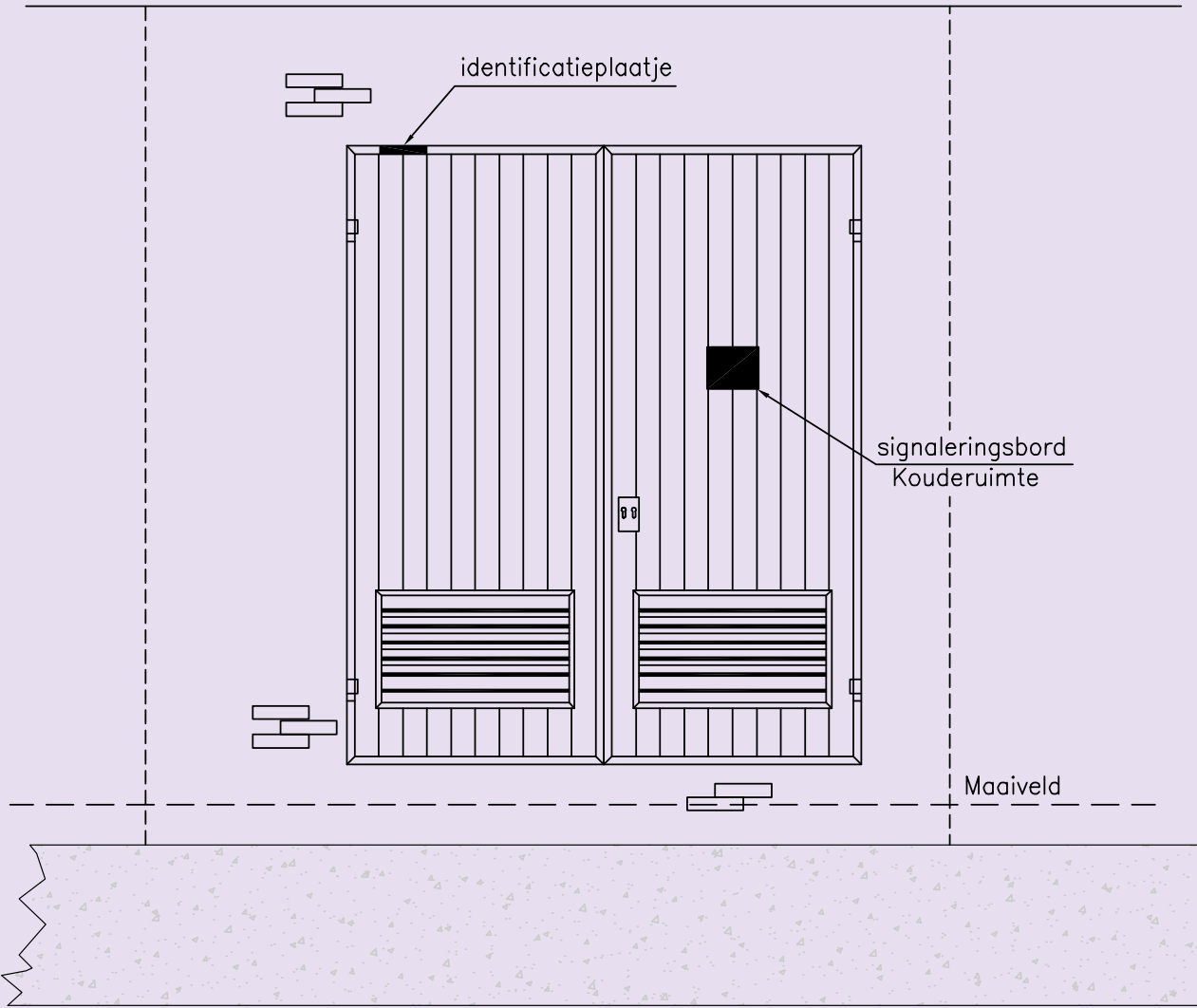
Voorbeeld van een ruimte voor afleverstation KAS DN80
