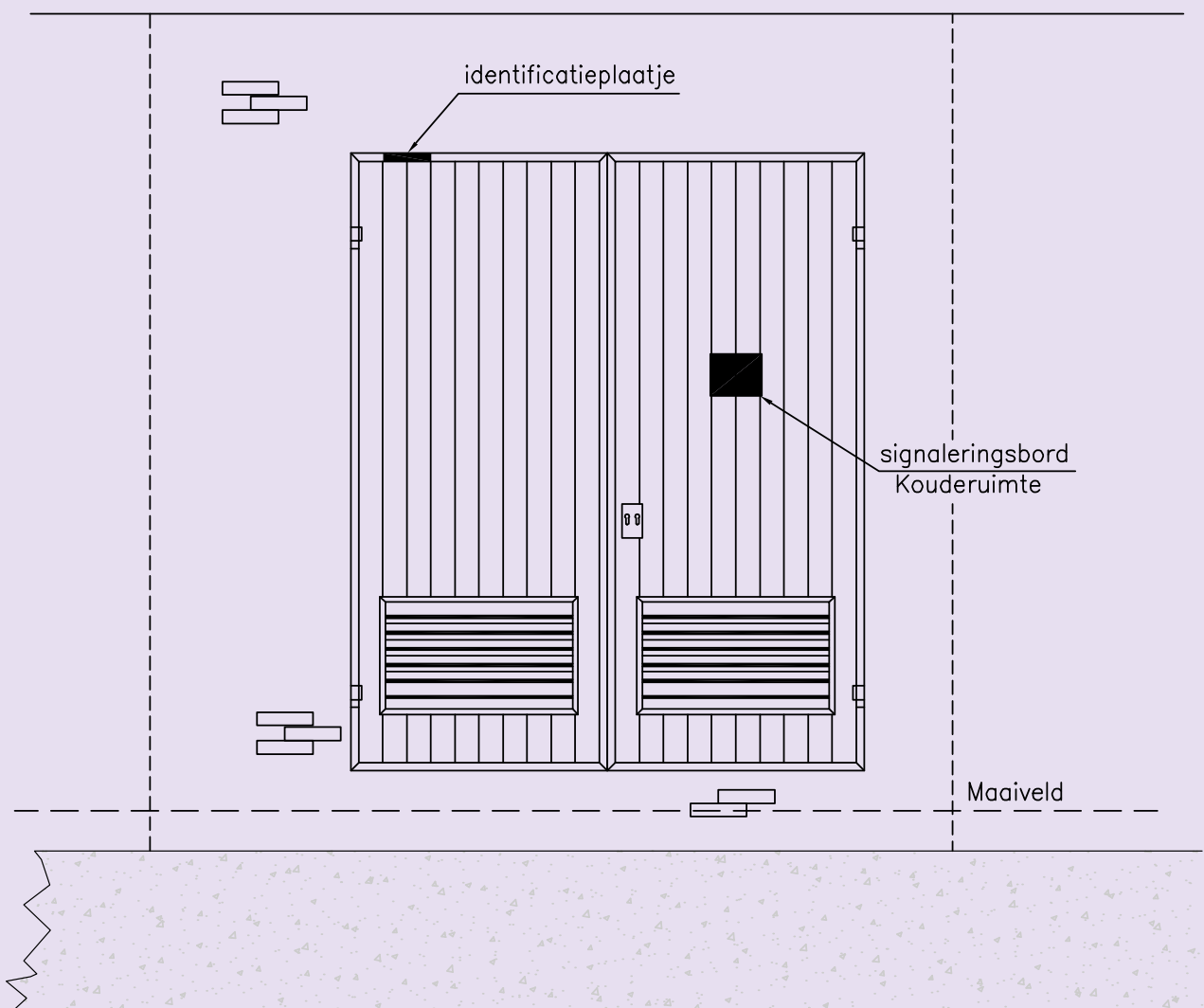
Vooraanzicht gevel (A-A)
