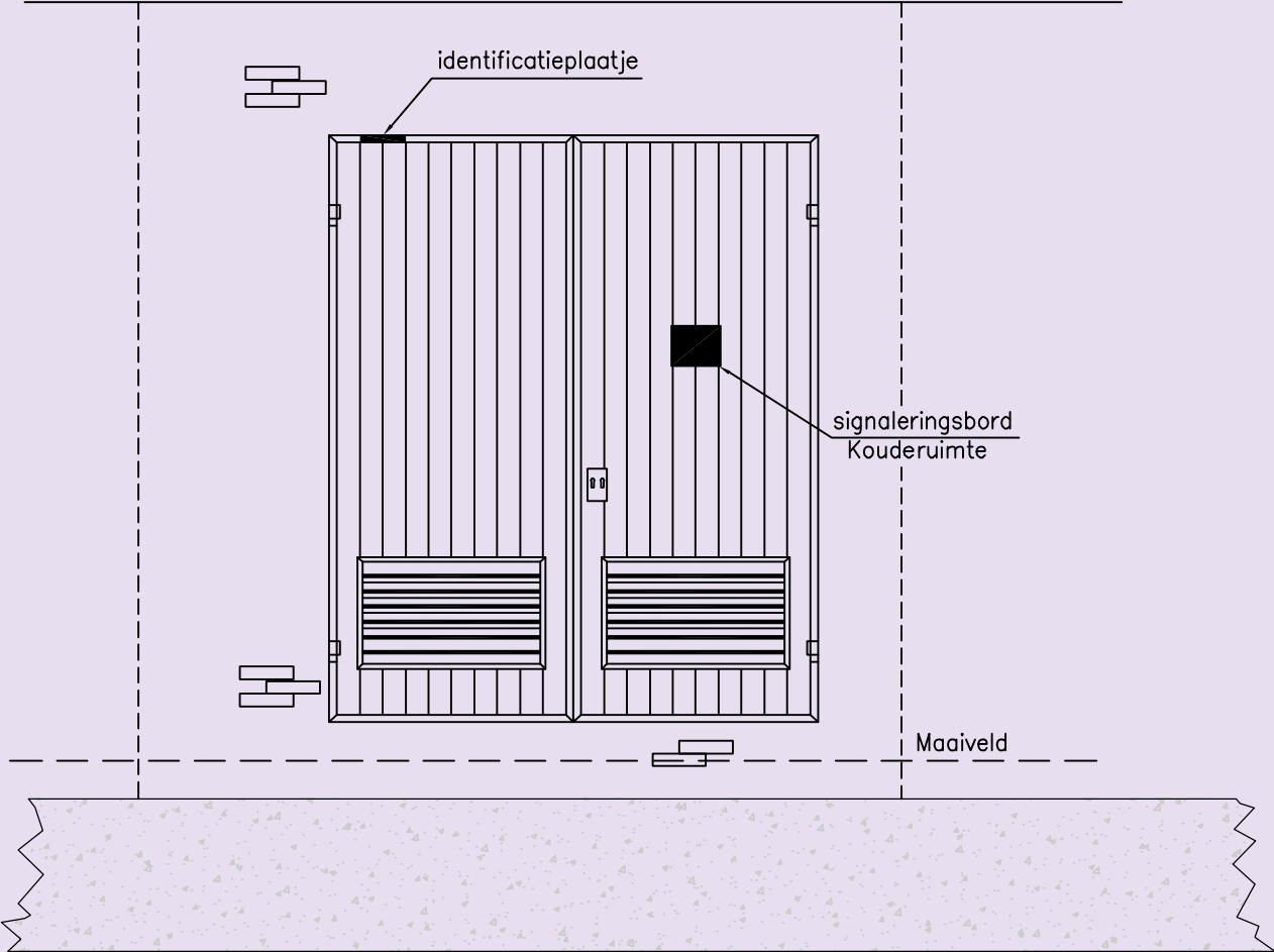
Vooranzicht gevel (A-A)
