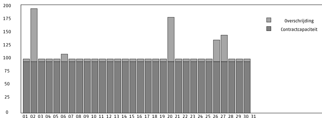
Gas Capaciteitoverschrijding per dag in m3/h - Overzicht per 2 september 2010
